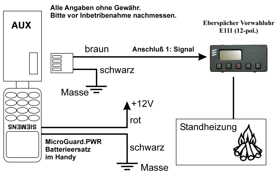
Abbildung 1: Schematische Darstellung des Anschlusses von Steuermodul und Standheizungssteuerung
